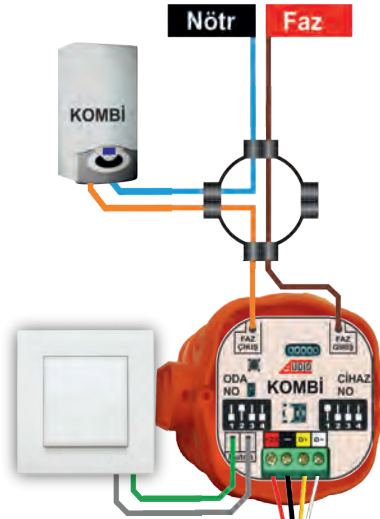
KOMBİ BAĞLANTISI
