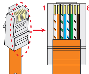
RJ-45 KABLO SIRALAMASI
