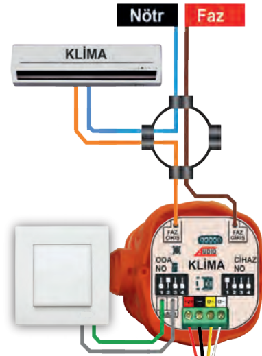
KLİMA BAĞLANTISI
