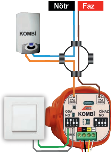
KOMBİ BAĞLANTISI
