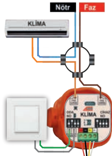
OTOMASYON KABLOSU (OK-4)
