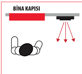
YANLIŞ MONTAJ
