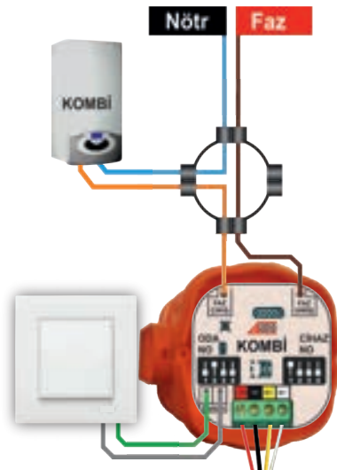
KOMBİ BAĞLANTISI
