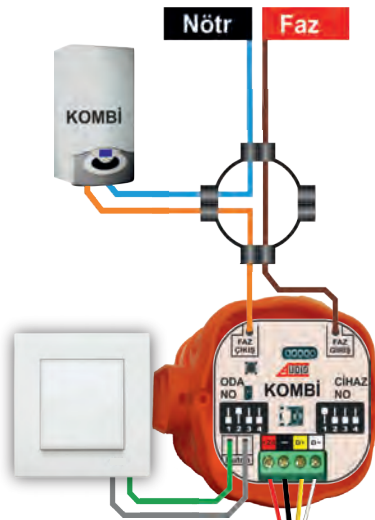
KOMBİ BAĞLANTISI
