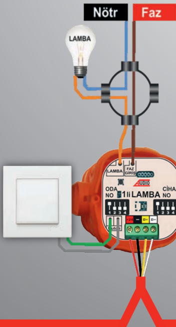
1'li LAMBA BAĞLANTISI
