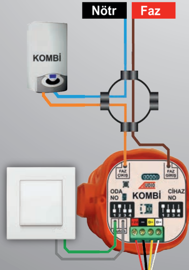
KOMBİ BAĞLANTISI
