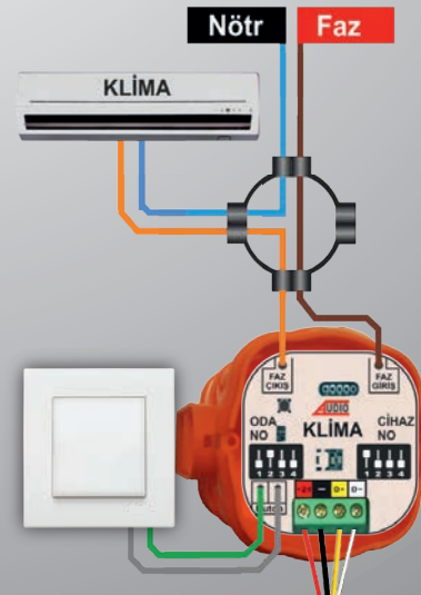
OTOMASYON KABLOSU(OK-4)
