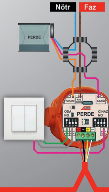
PERDE BAĞLANTISI
