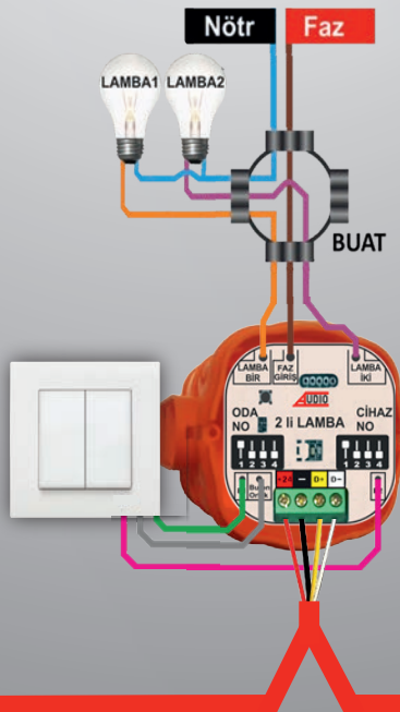
2'li LAMBA BAĞLANTISI
