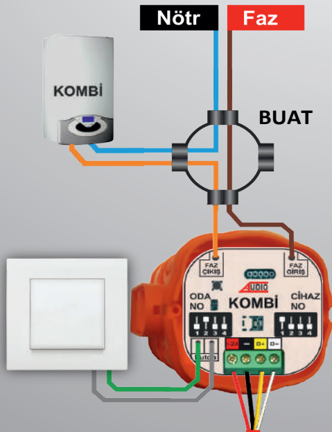
KOMBİ BAĞLANTISI
