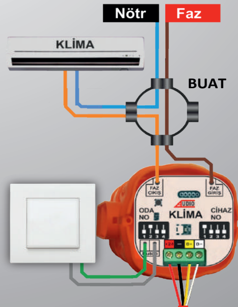
OTOMASYON KABLOSU(OK-4)
