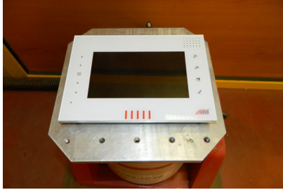
VİBRASYON TESTİ
